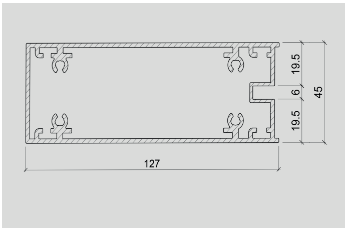
Abschlussprofil
