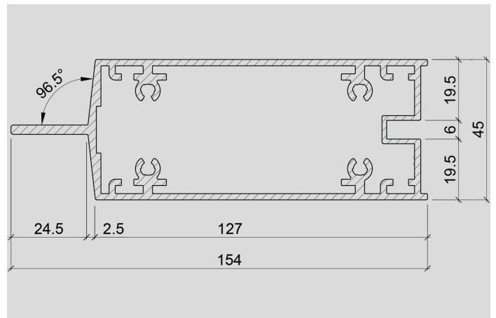
Basisprofil
